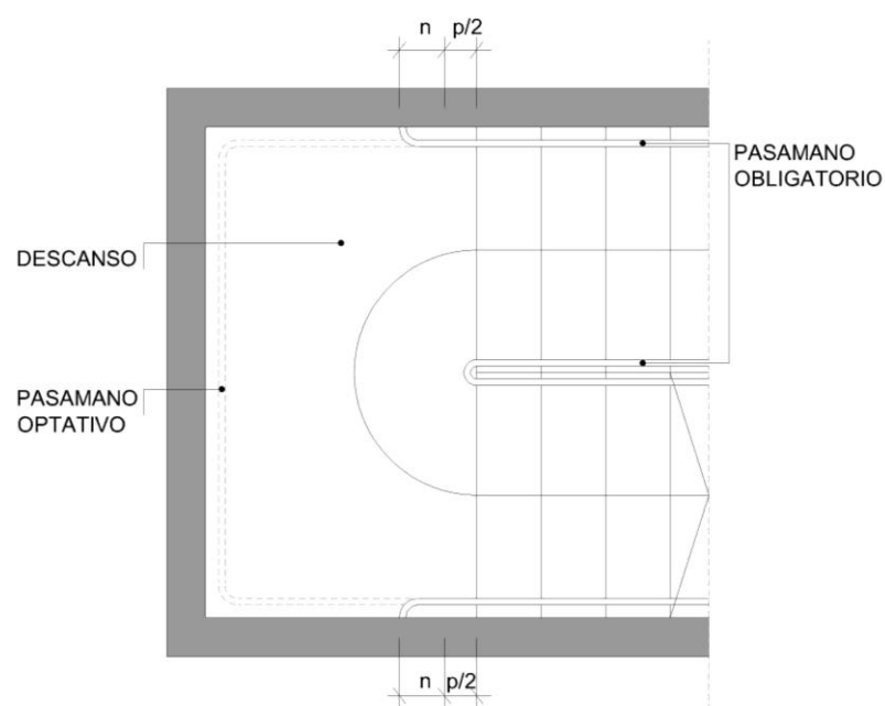
PLANTA DE TRAMO DE ESCALERA CON DESCANSO Y GIRO A 180°
