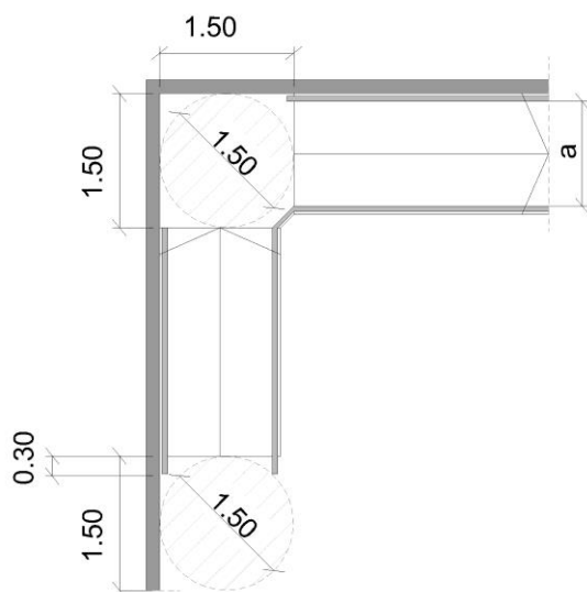
a) GIRO A 90°
