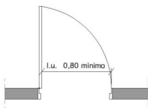
1. HOJA CON BISAGRA, FICHA O POMELO DE EJE VERTICAL
